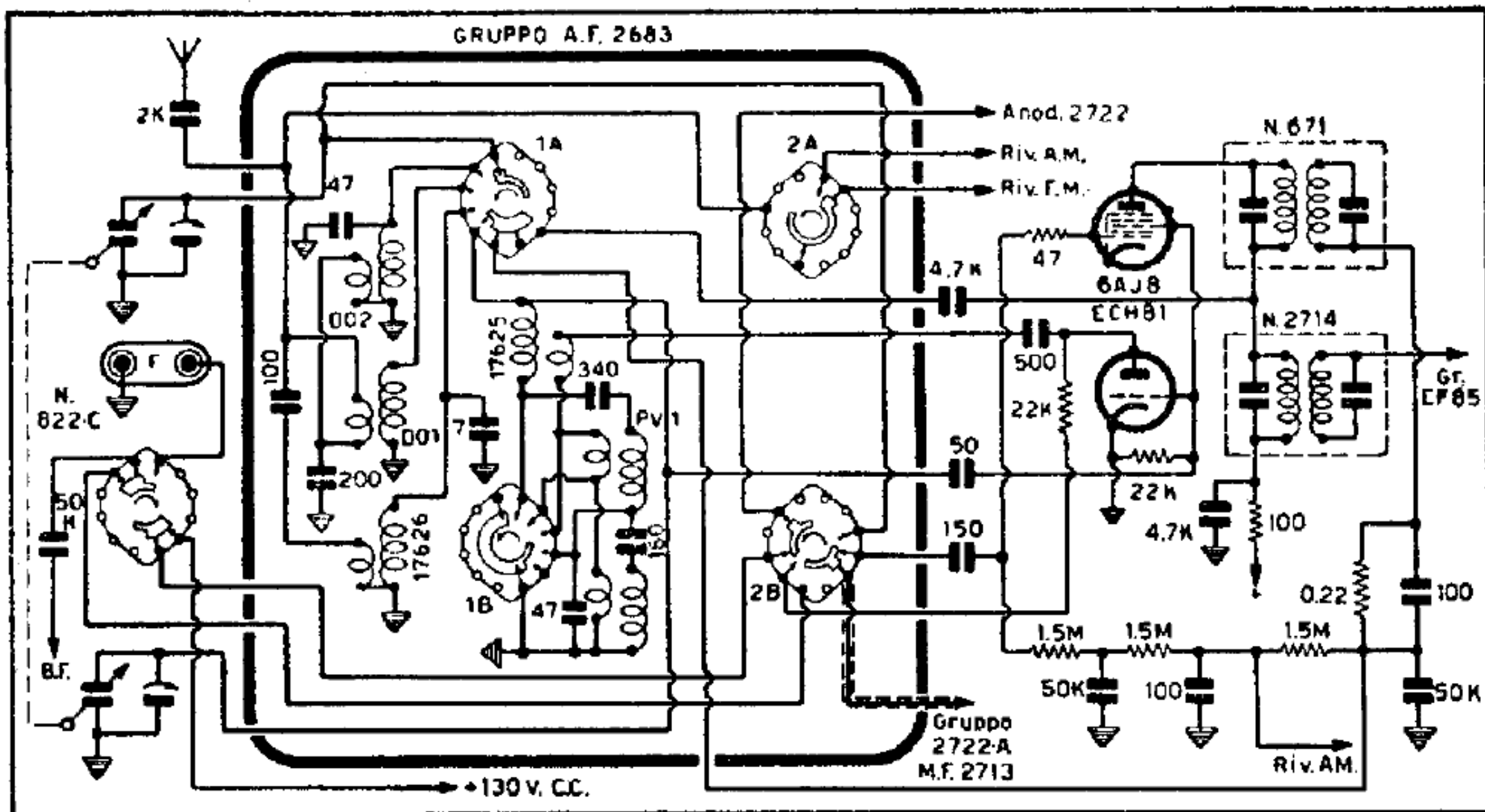
Flange viste dal lato lastiera supporto bobine in basso, posizione F.M.
